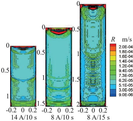
图5 不同磁场条件下的 Ti-1023 铸锭凝固速率分布
