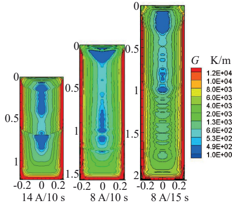
图4 不同磁场条件下的 Ti-1023 铸锭温度梯度分布
