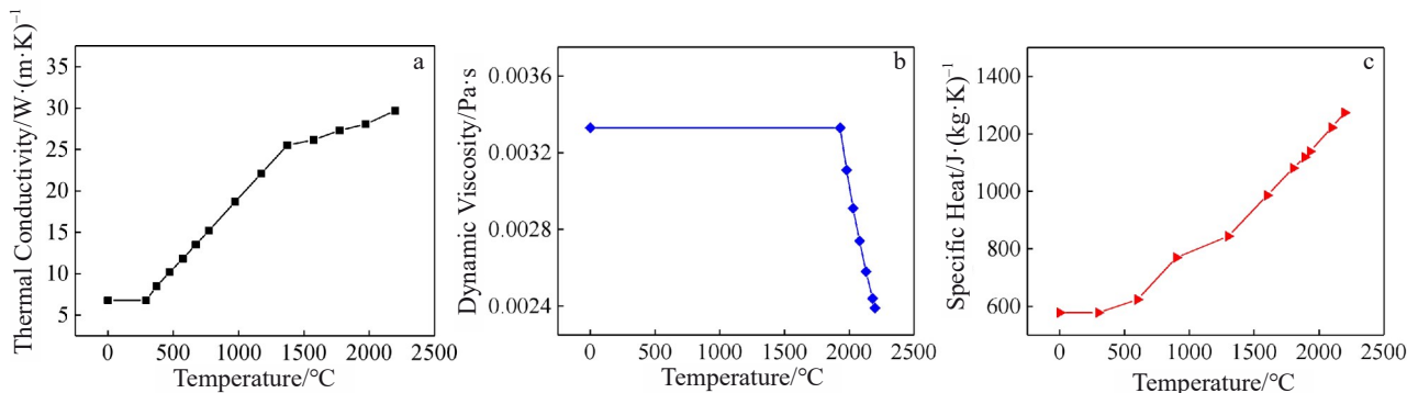
图 2 Ti-1023 合金变温物性参数
